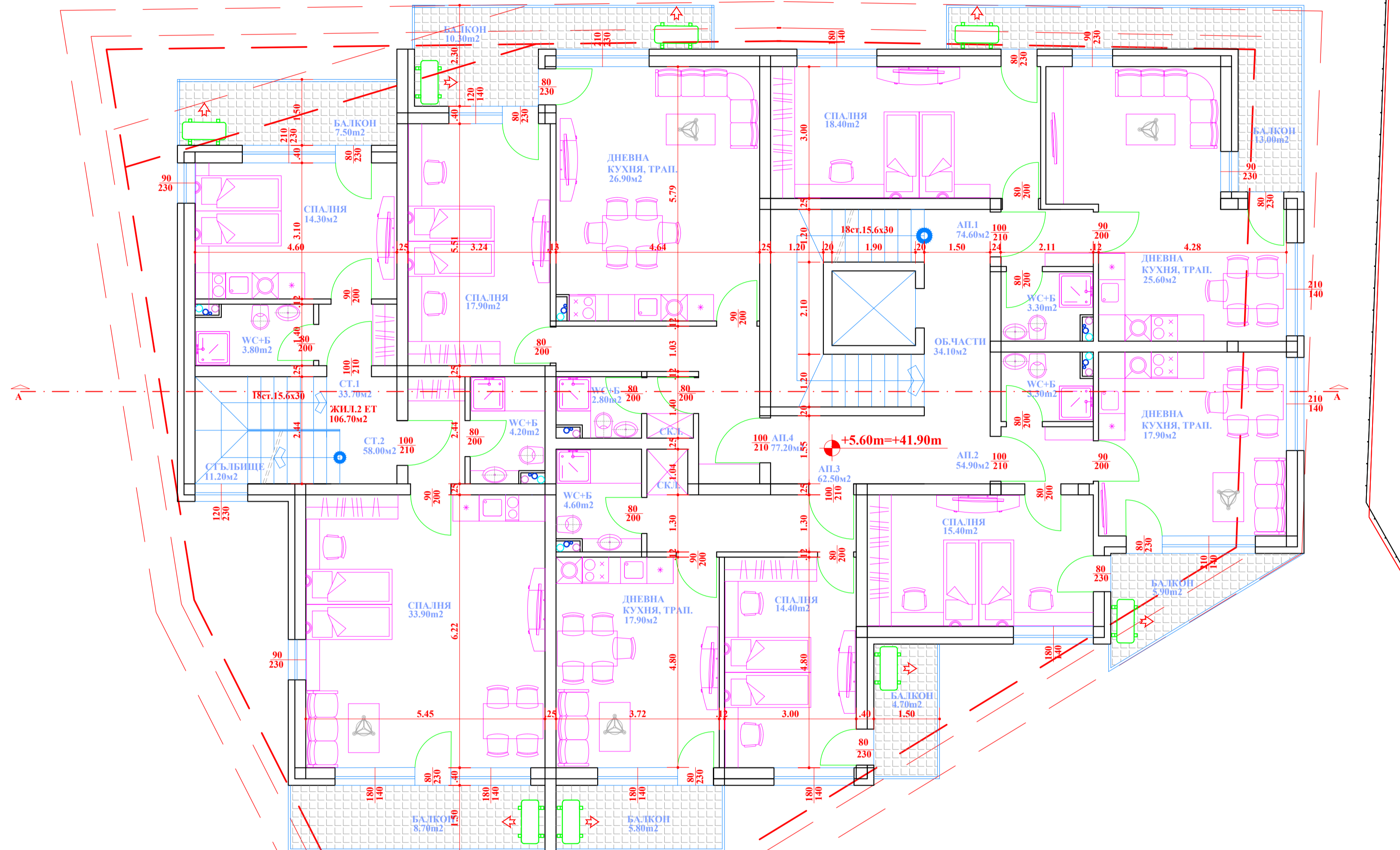
РАЗПРЕДЕЛЕНИЕ 2 ЕТАЖ НА КОТА +5.60m - +41.90m ЗАСТРОЕНА ПЛОЩ 410.10 m 2
